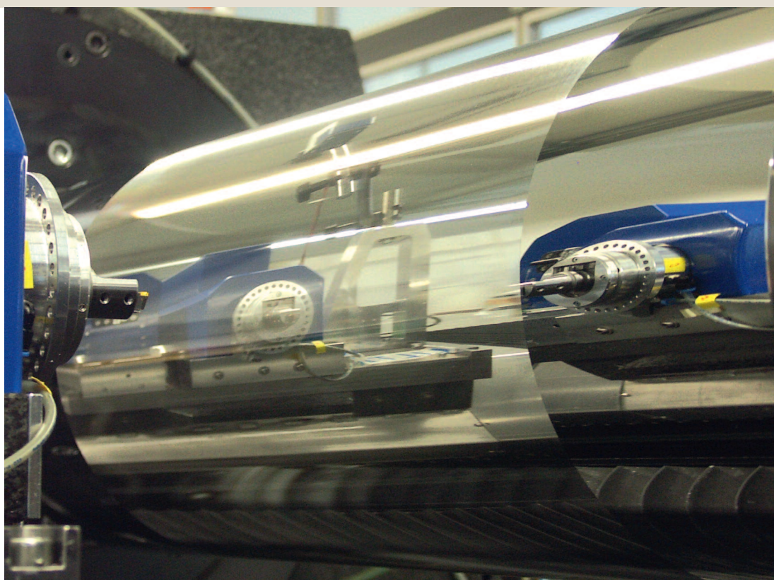
Bild 1. Bearbeitung einer Prägewalze (Nickelphosphor) mit einer »LT Ultra DTM2300«
