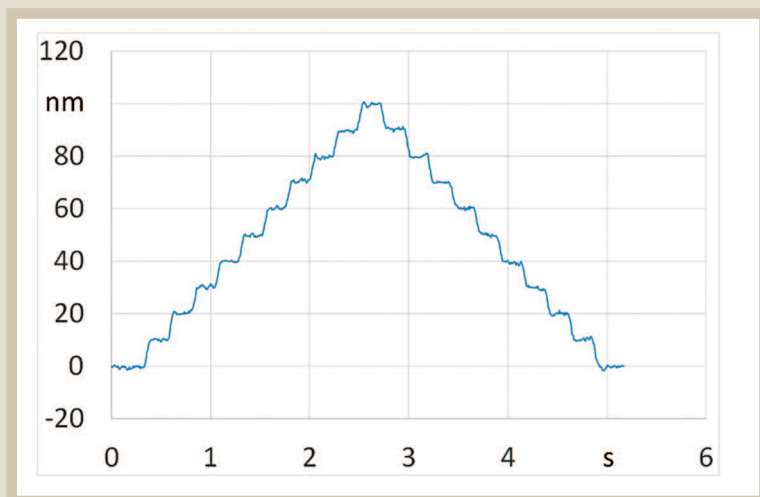
Bild 2. Treppenstufentest der X-Achse einer MMC-900H-Ultrapräzisionsfräsmaschine von LT Ultra
